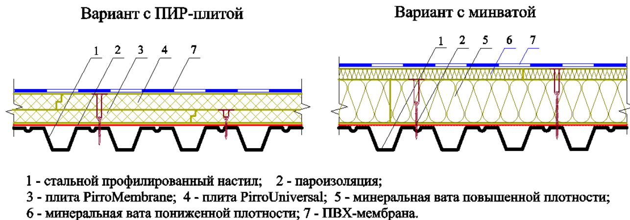
Рис. 1 Варианты конструкции кровельного пирога для PIR-плиты и минеральной ваты
